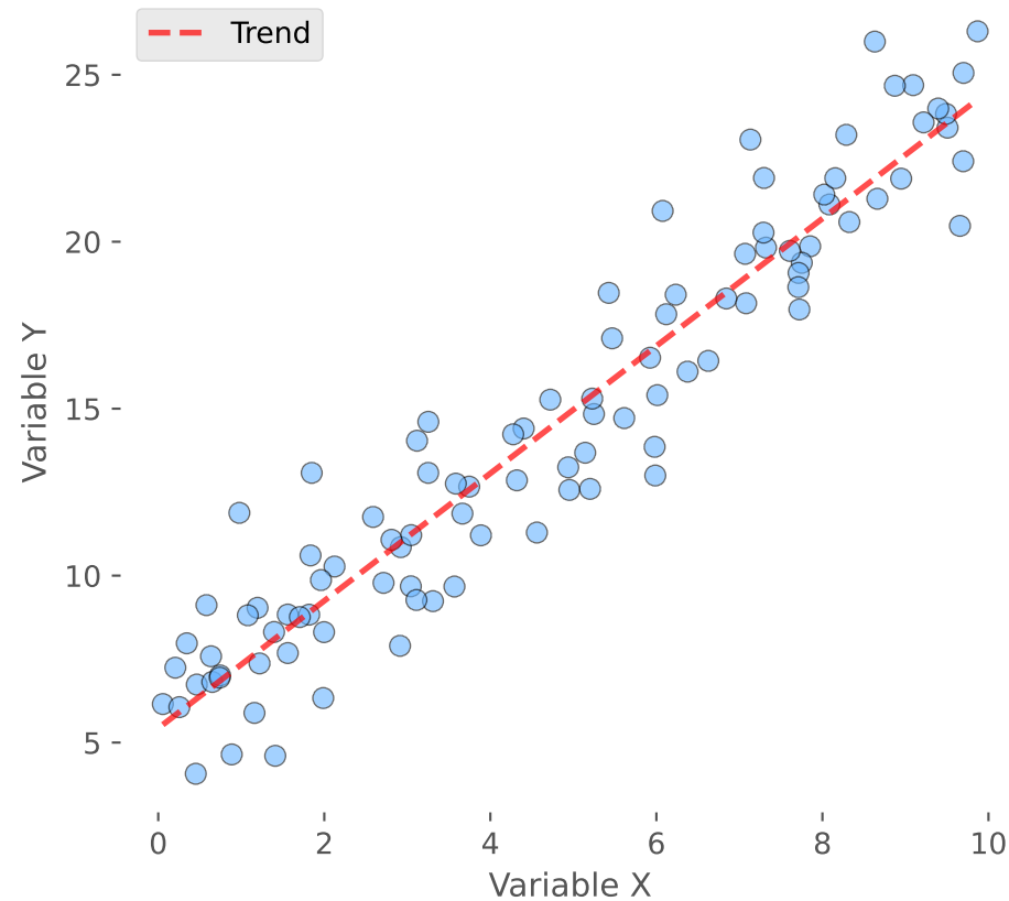
Positive Korrelation (X steigt → Y steigt)
