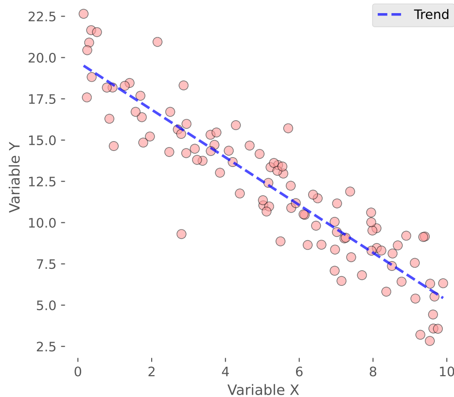
Negative Korrelation (X steigt → Y sinkt)
