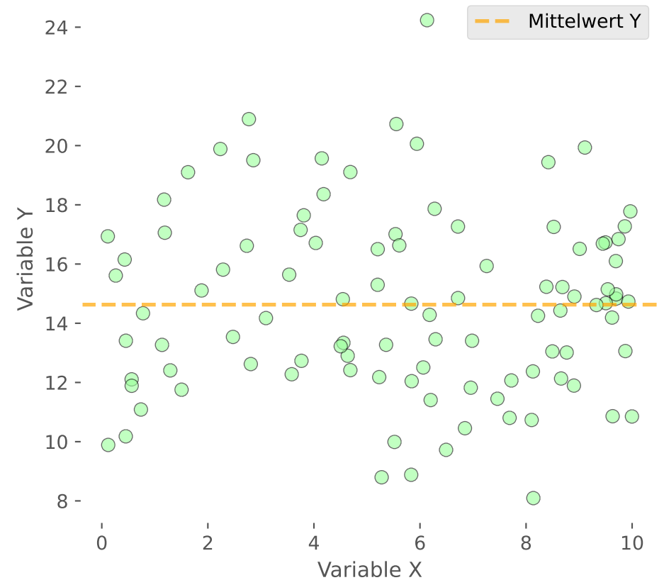
Keine Korrelation (kein systematischer Zusammenhang)
